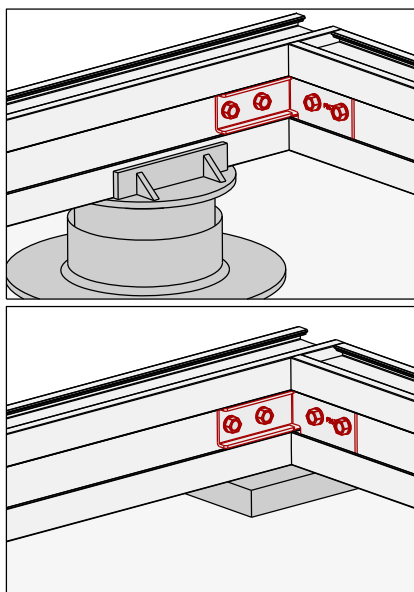
connection d'angle
