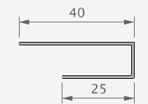
P 109 U-afwerkingsprofiel
